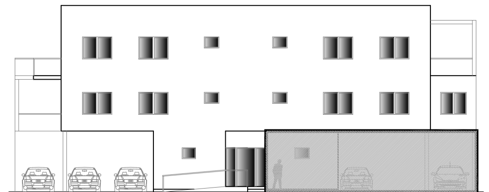
STAN D2 Sjeveroistočno pročelje
