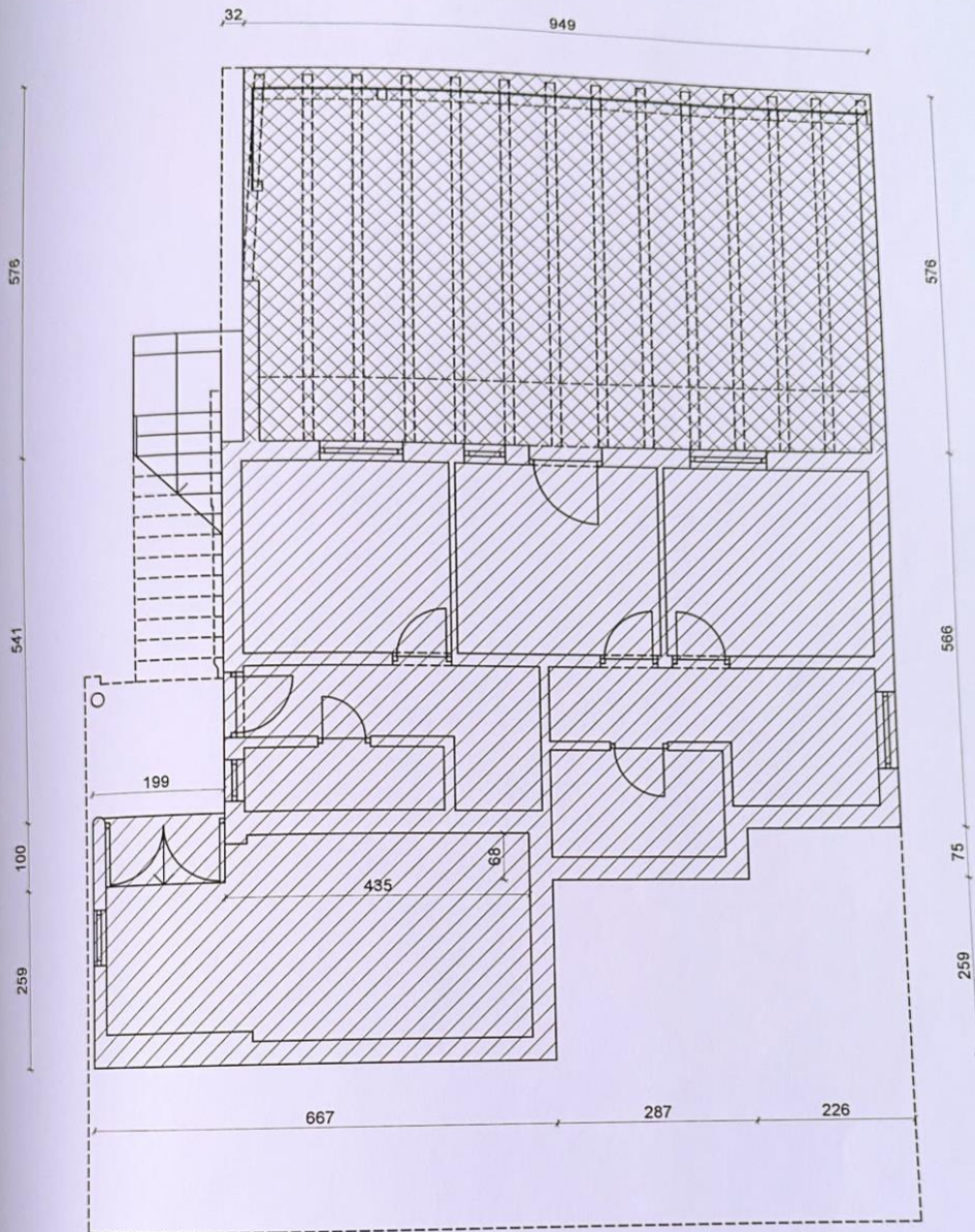
TLOCRT PRIZEMLJA
