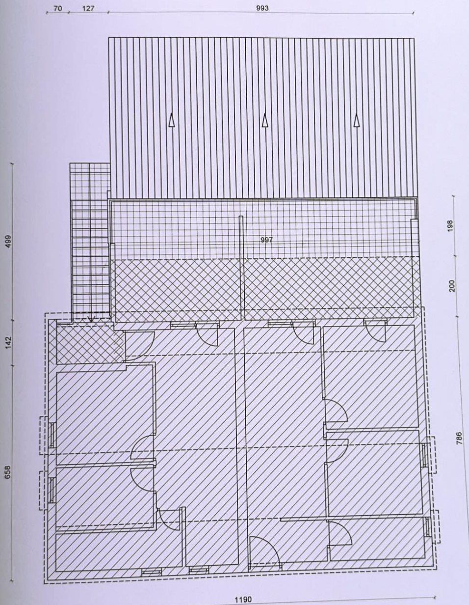
TLOCRT KATA
