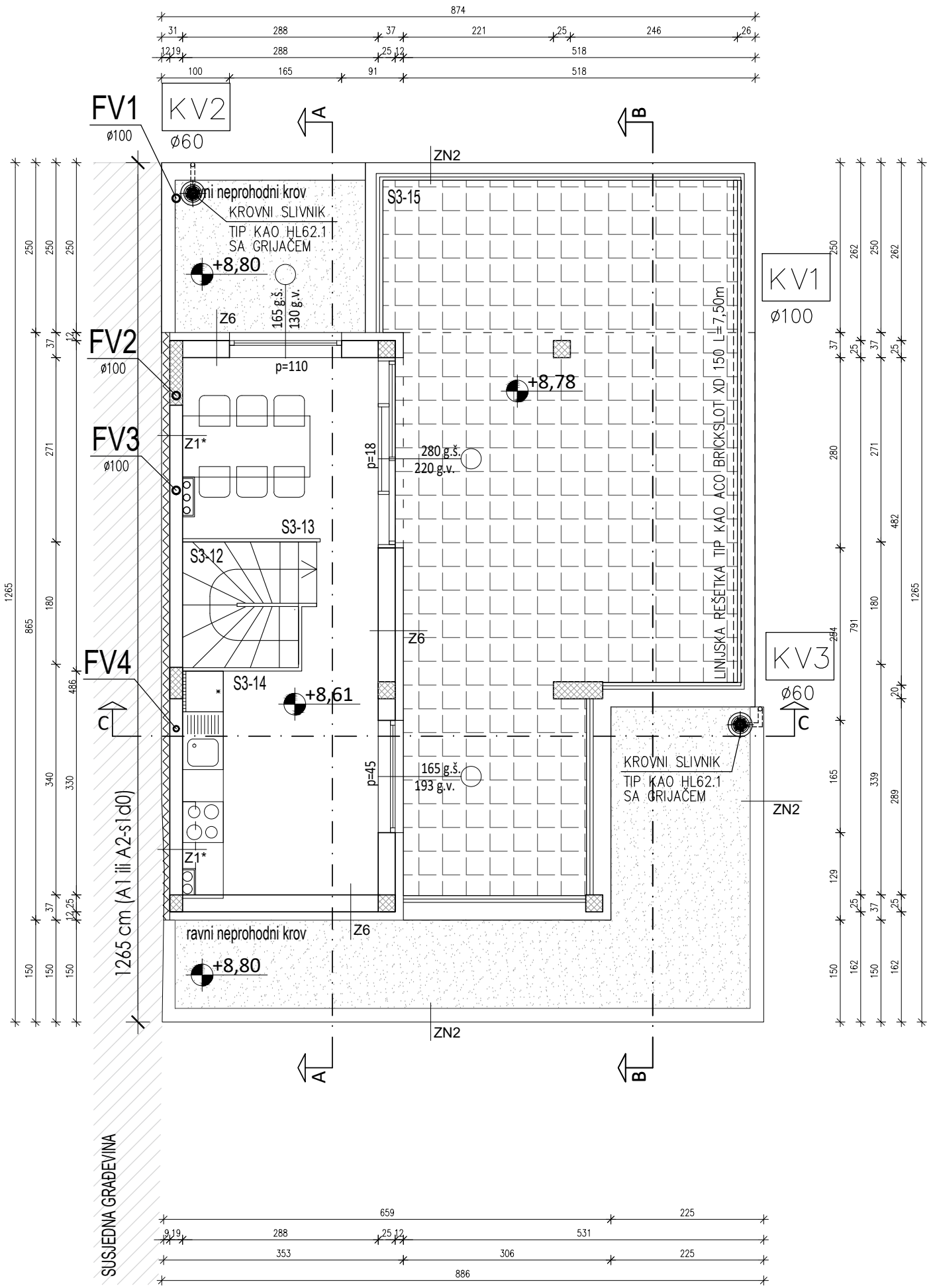
TLOCRT UVUČENOG KATA
