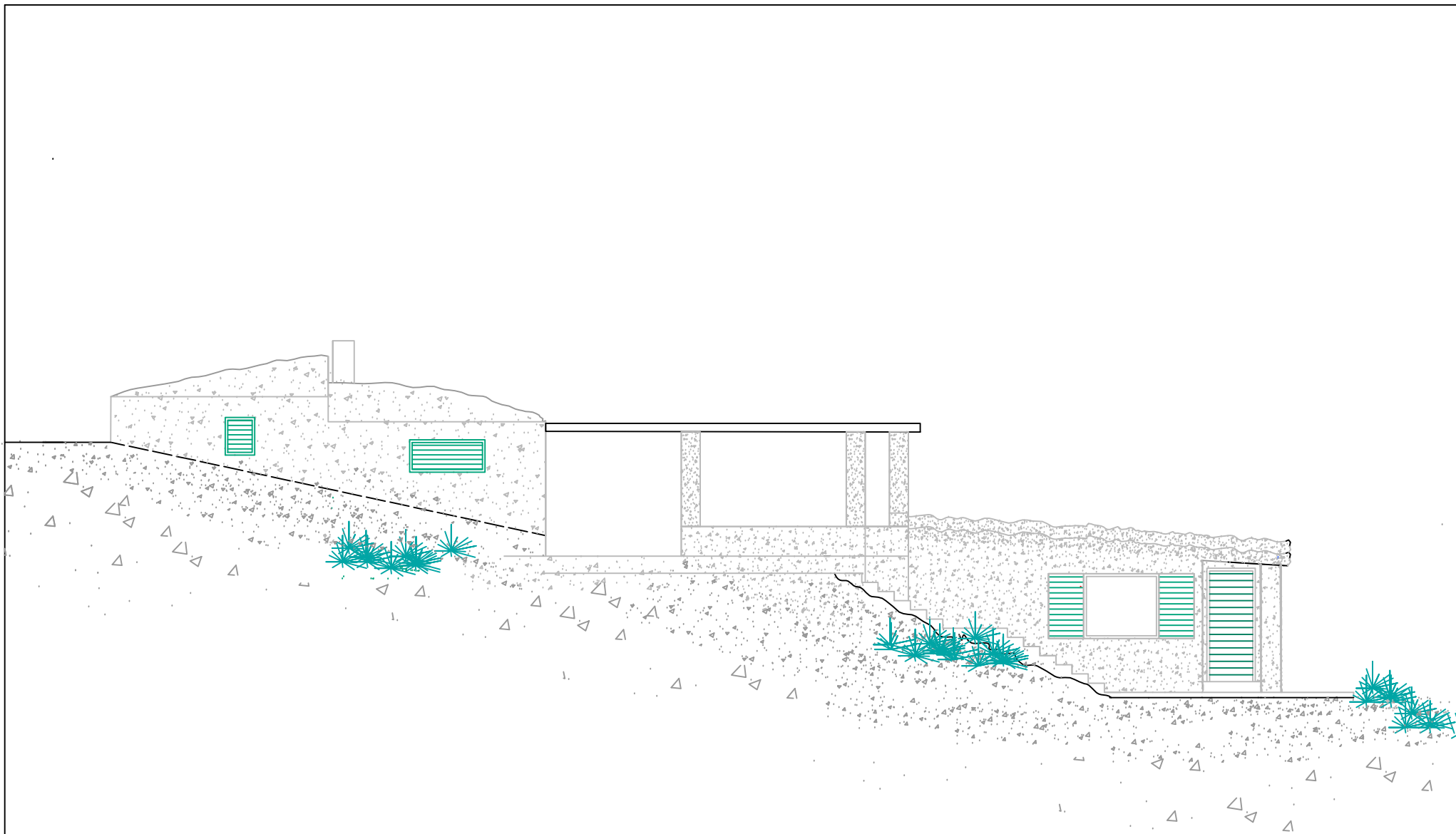
SJEVERNA FASADA
