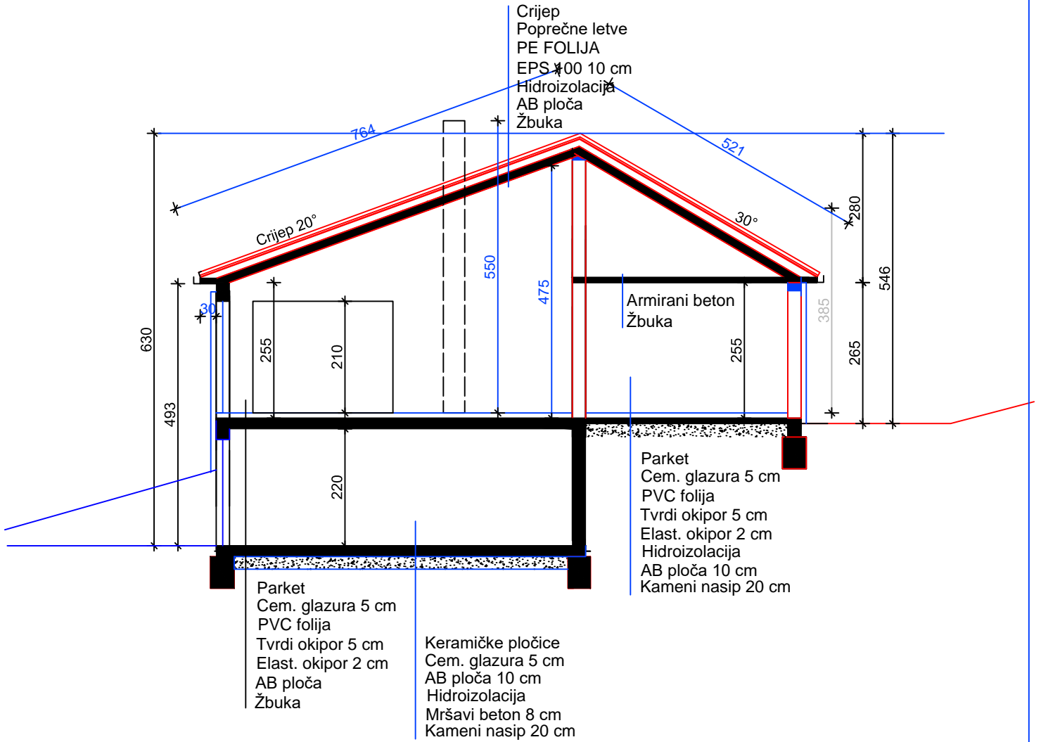
PRESJEK A-A
