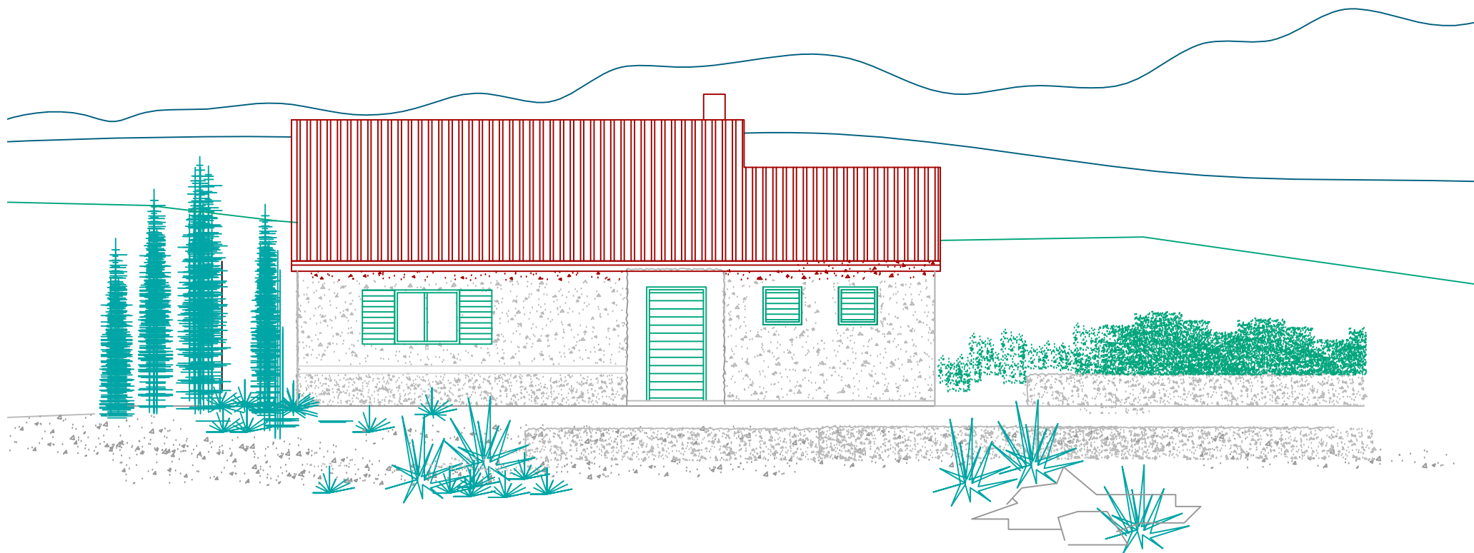
ZAPADNA FASADA
