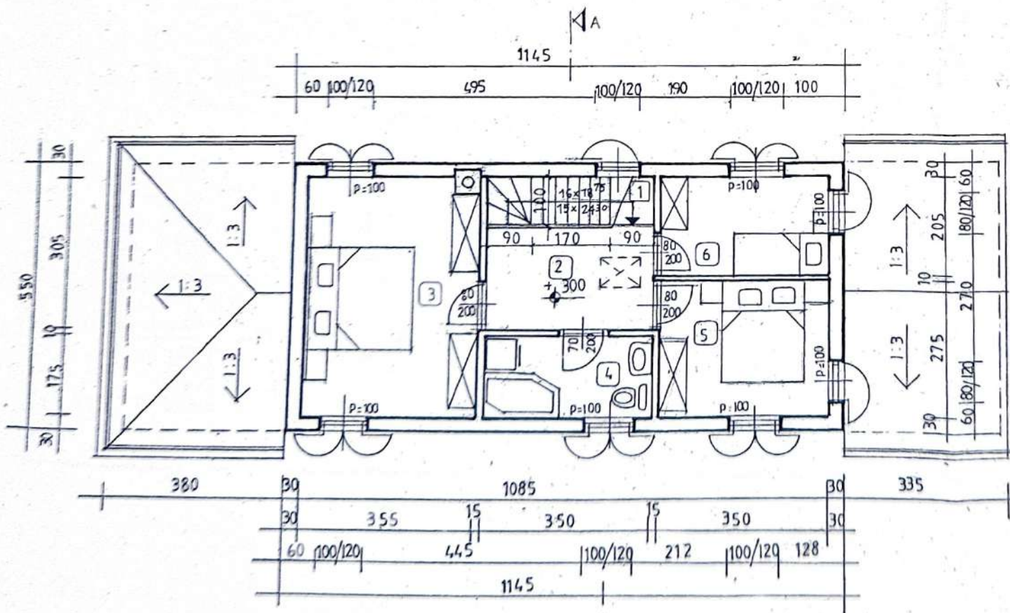
tlocrt kata 1:100
