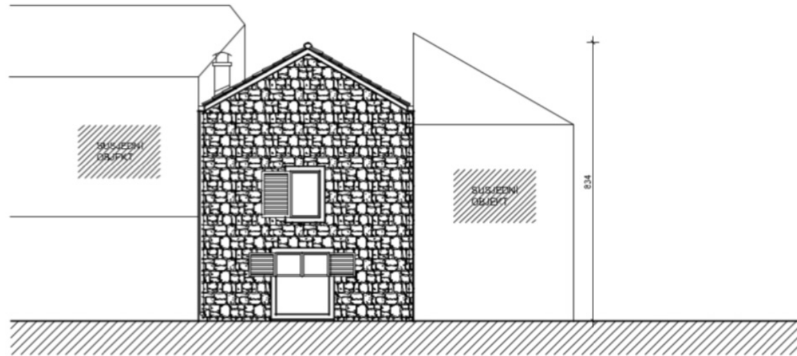
ZAPADNO PROČELJE Mjerilo 1:100 Novoprojektirano stanje
