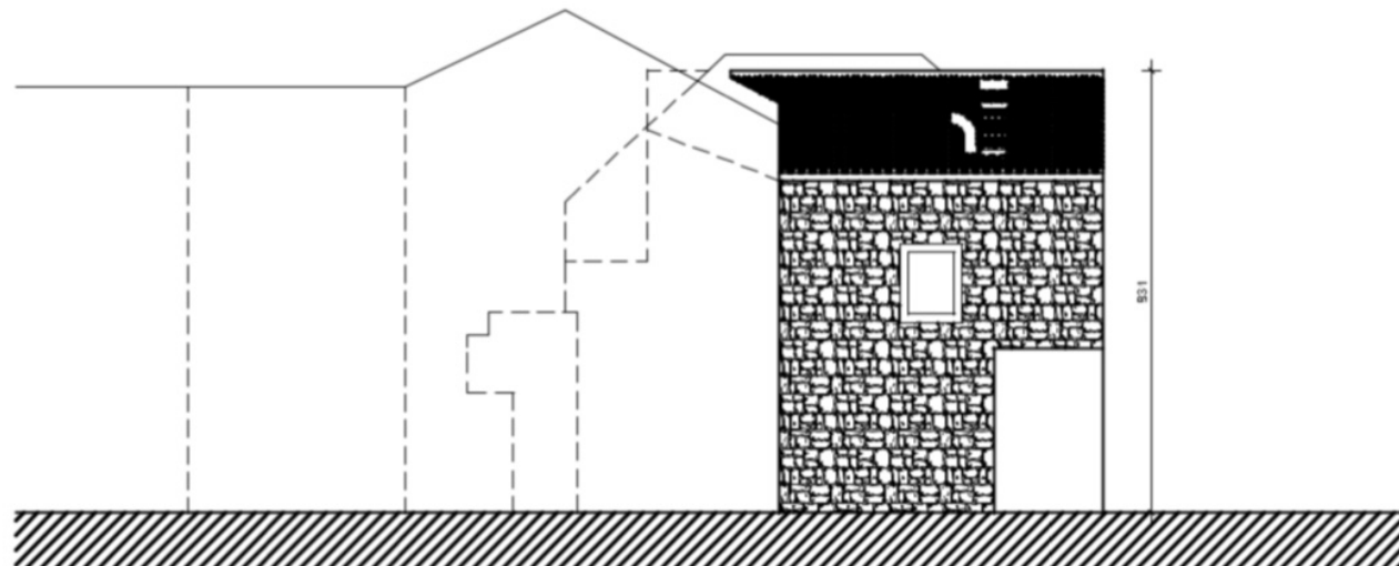
ZAPADNO PROČELJE Mjerilo 1:100 Novoprojektirano stanje
