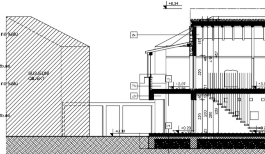
PRESJEK A-A Mjerilo 1:100 Novoprojektirano stanje
