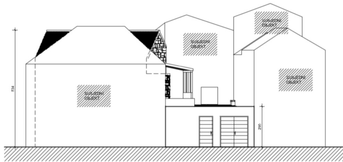
ISTOČNO PROČELJE Mjerilo 1:10 Novoprojektirano stanj
