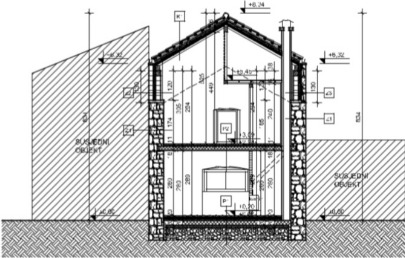
PRESJEK A-A Mjerilo 1:100 Novoprojektirano stanje
